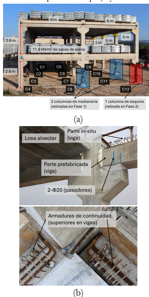
Figura 1. (a) Disposición y geometrías clave de la probeta prefabricada construida al efecto (los pilares que deben retirarse también están resaltados en colores rojo y azul); (b) La conexión viga-pilar de resistencia parcial.
