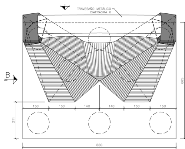
Figura 4. Planta de Pila
