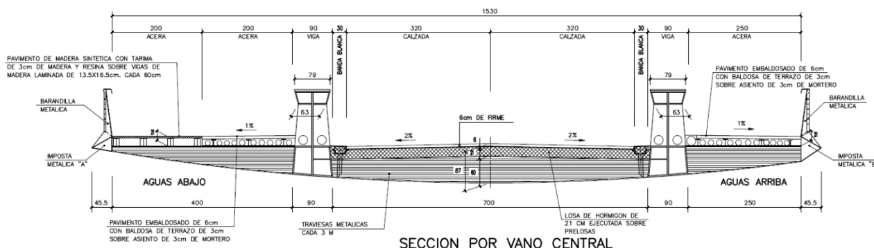
Figura 2. Sección tipo
