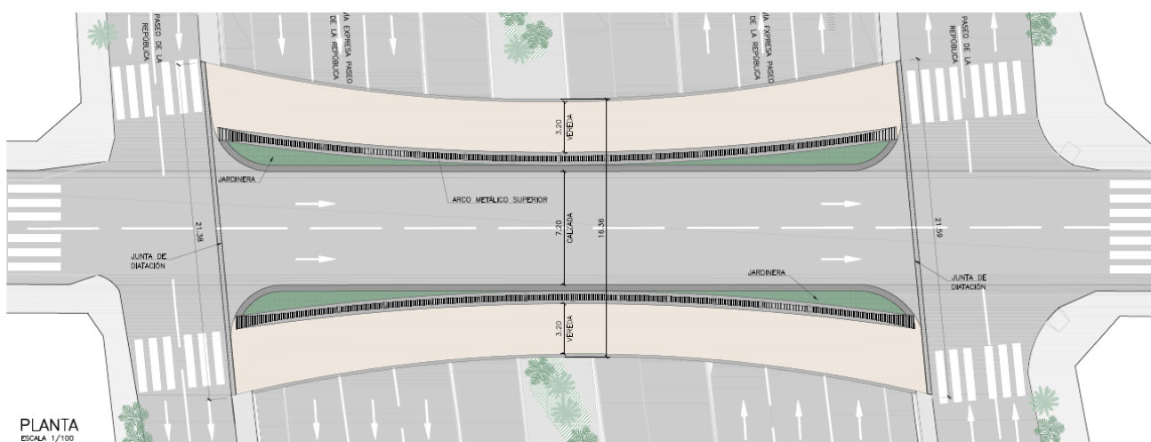
Figura 8. Alzado y planta del Puente Leoncio Prado.
