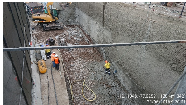
Figura 11. Sostenimiento provisional.
