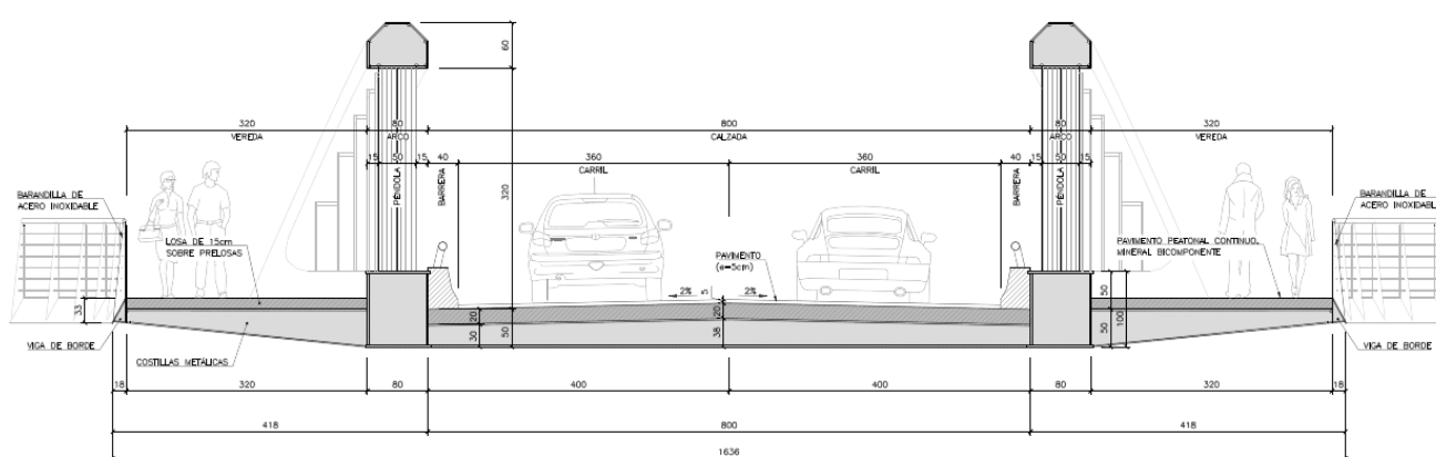
Figura 9. Sección transversal del Puente Leoncio Prado.
