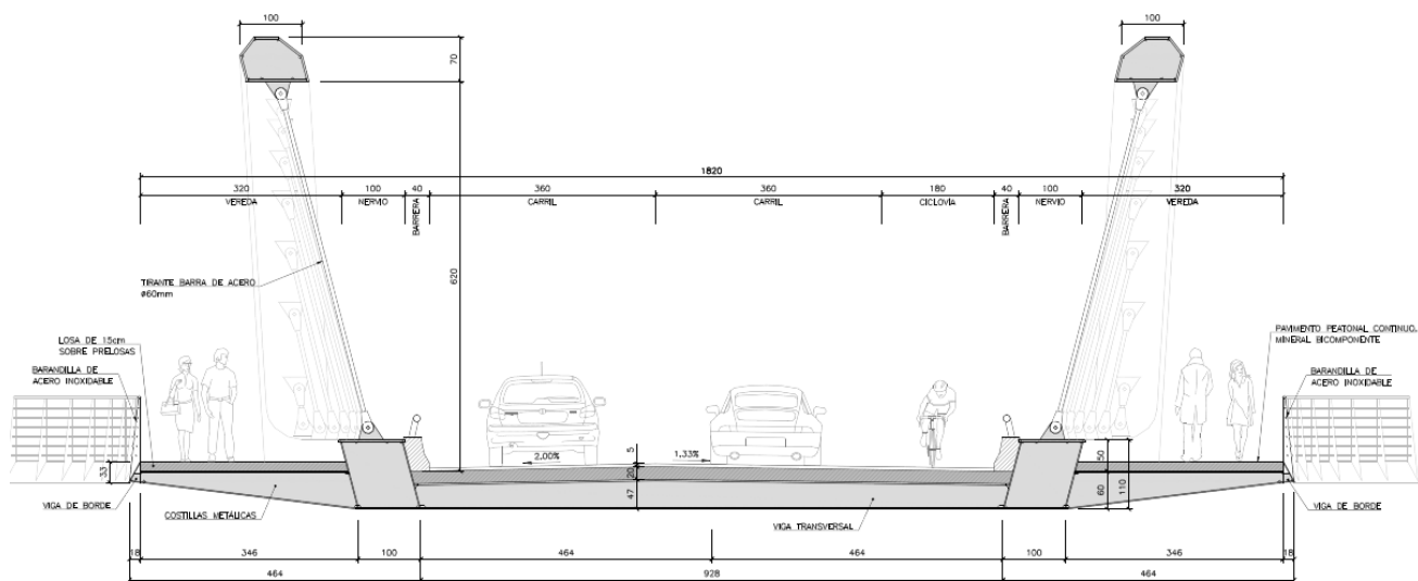
Figura 7. Sección transversal del Puente Junín.
