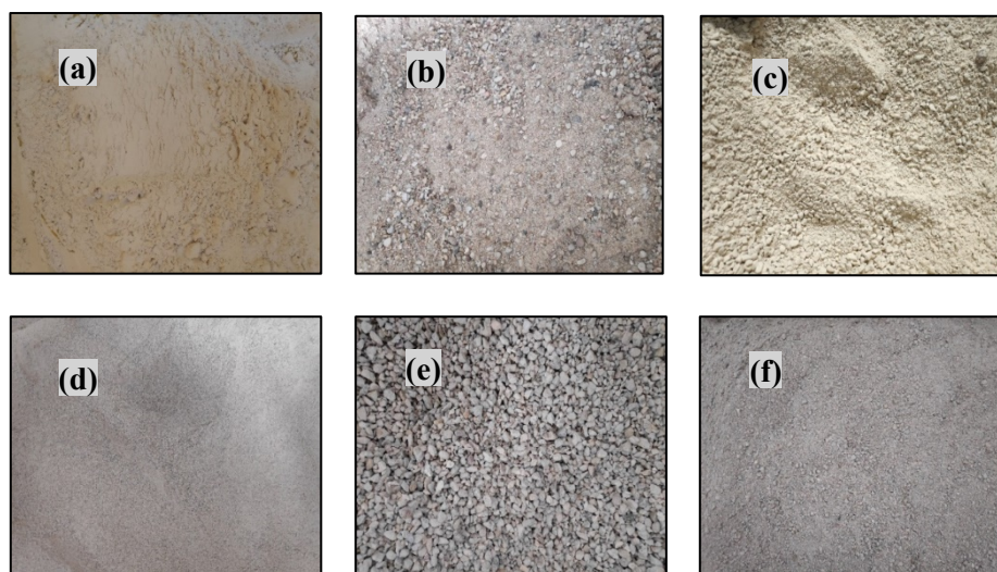
Figura 2. Áridos utilizados. a-Filler calizo (<math><0.063\text{ mm}</math>). b-Arena sílicea (0/4 mm). c-Arena caliza (0/4 mm). d-Arena caliza (0/1.2 mm). e- RCA grueso (4/12.5 mm). f-RCA fino (0/4mm)
