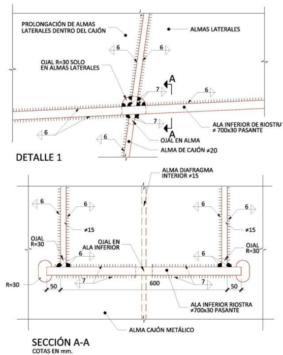
Figura 10. Detalle de intersección de ala inferior de riostra nº 1 con el alma de cajón metálico.
