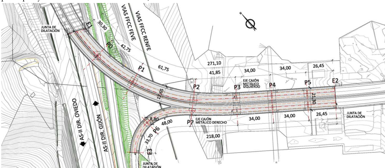
Figura 3. Planta general del viaducto.
