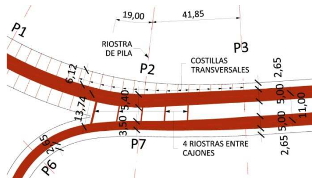
Figura 8. Esquema transición de cajones metálicos.
