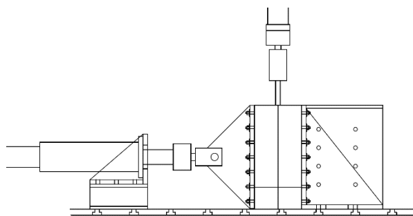
Figura 7: Setup ensayos de tracción
