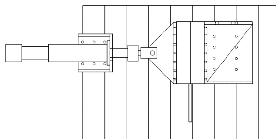
Figura 8: Montaje ensayo de cortante, vista en planta
