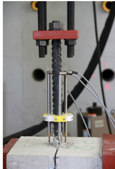
Figura 15: Instrumentación del anclaje
